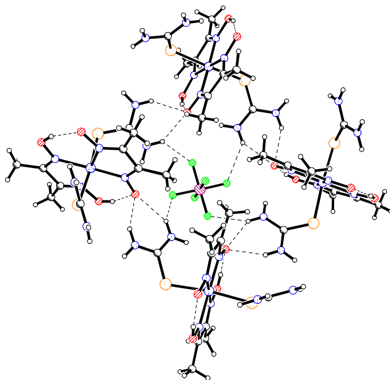
Fig. 2. Patru cationi complecși formează “tunele” ocupate de anionii \text{PF}_6^-
