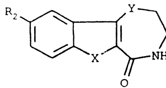
2,3-dihidro-9-metoxi-(1)benzotieno[2,3-f]-1,4-tiazepin-5(4H)-onă
